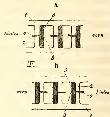
Schema der Bildung der Scheidewände: 1) sehnige Haut, 2) Scheidewand, 3) pseudoelektrische Platte, 4) Nerv des einzelnen Plättchens, 5) Ausbreitung desselben.
